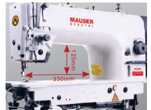
宽大的操作空间 Large arm clearance
