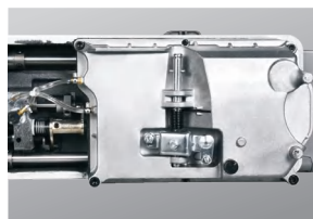
双动刀剪线设计，在机针正下方剪断缝线，已申报专利
